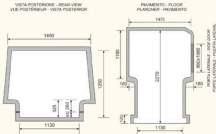
PORTALE POSTERIORE CON PORTE SUPPLEMENTARI (OPTIONAL) REAR DOOR FRAME WITH SUPPLEMENTARY DOORS (OPTIONAL) PORTAL POSTÉRIEUR AVEC PORTES SUPPLÉMENTAIRES (OPTIONAL) PORTON TRASERO CON PUERTAS SUPLEMENTARIAS (OPCIONAL)
